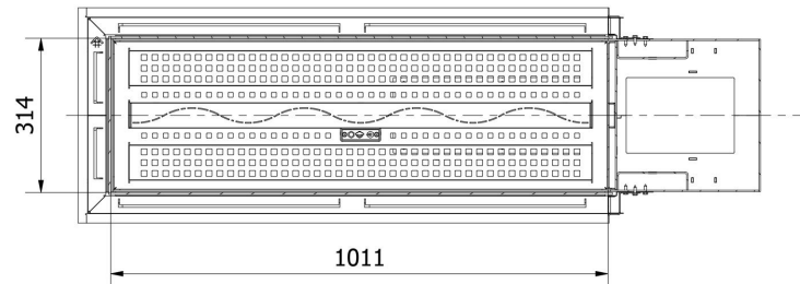
B-B ( 1 : 10 )
