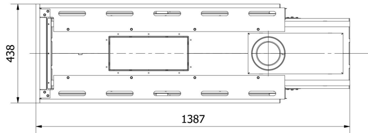
B-B ( 1 : 10 )
