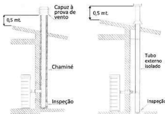
Fig. 2: ligação à chaminé Fig. 3: ligação a um tubo externo com tubo isolado ou parede dupla
