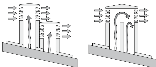
Fig. 5: caratteristiche del comignolo
